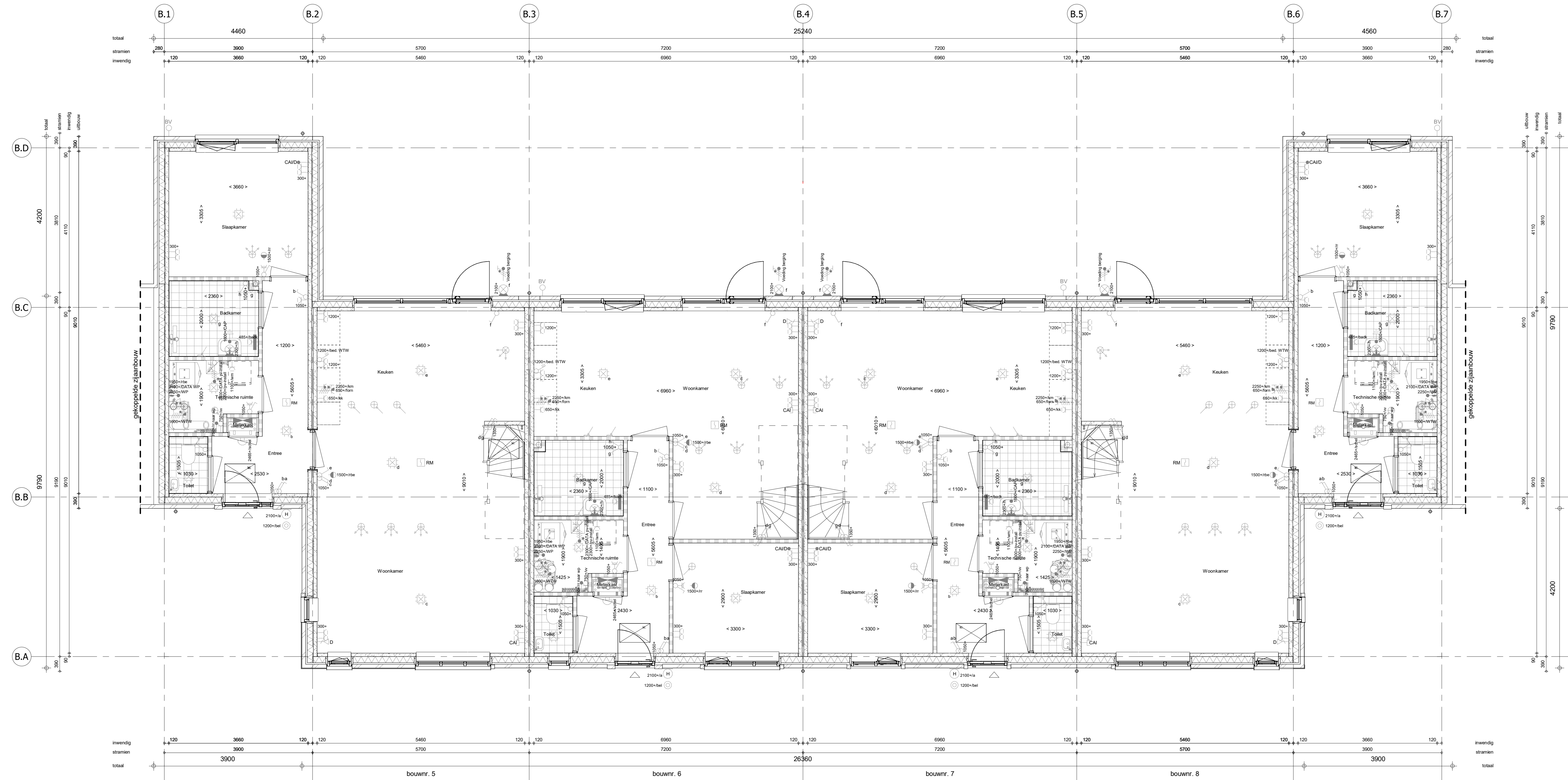
Begane grond 1 : 50
