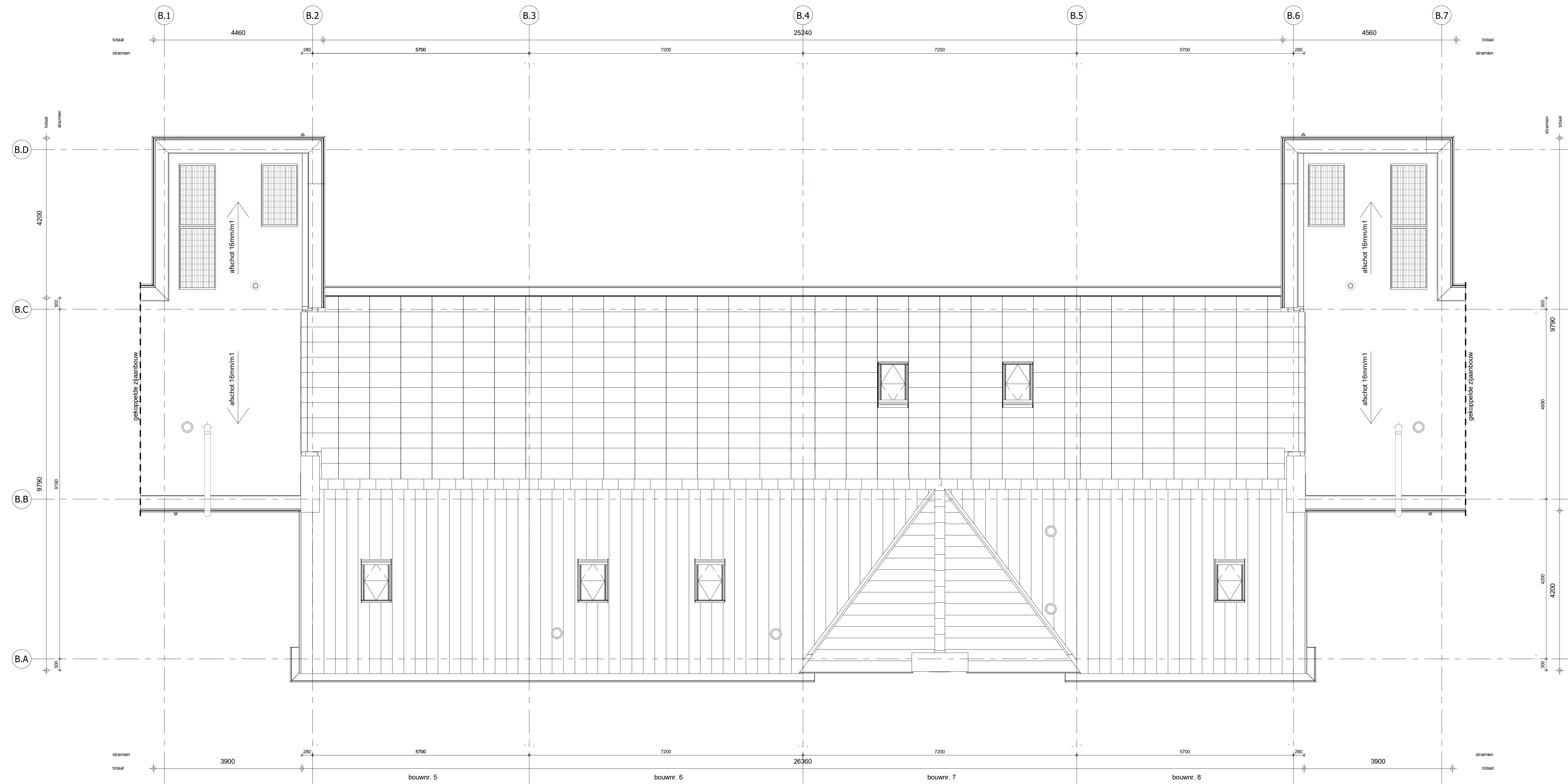
Dakaanzicht 1 : 50
