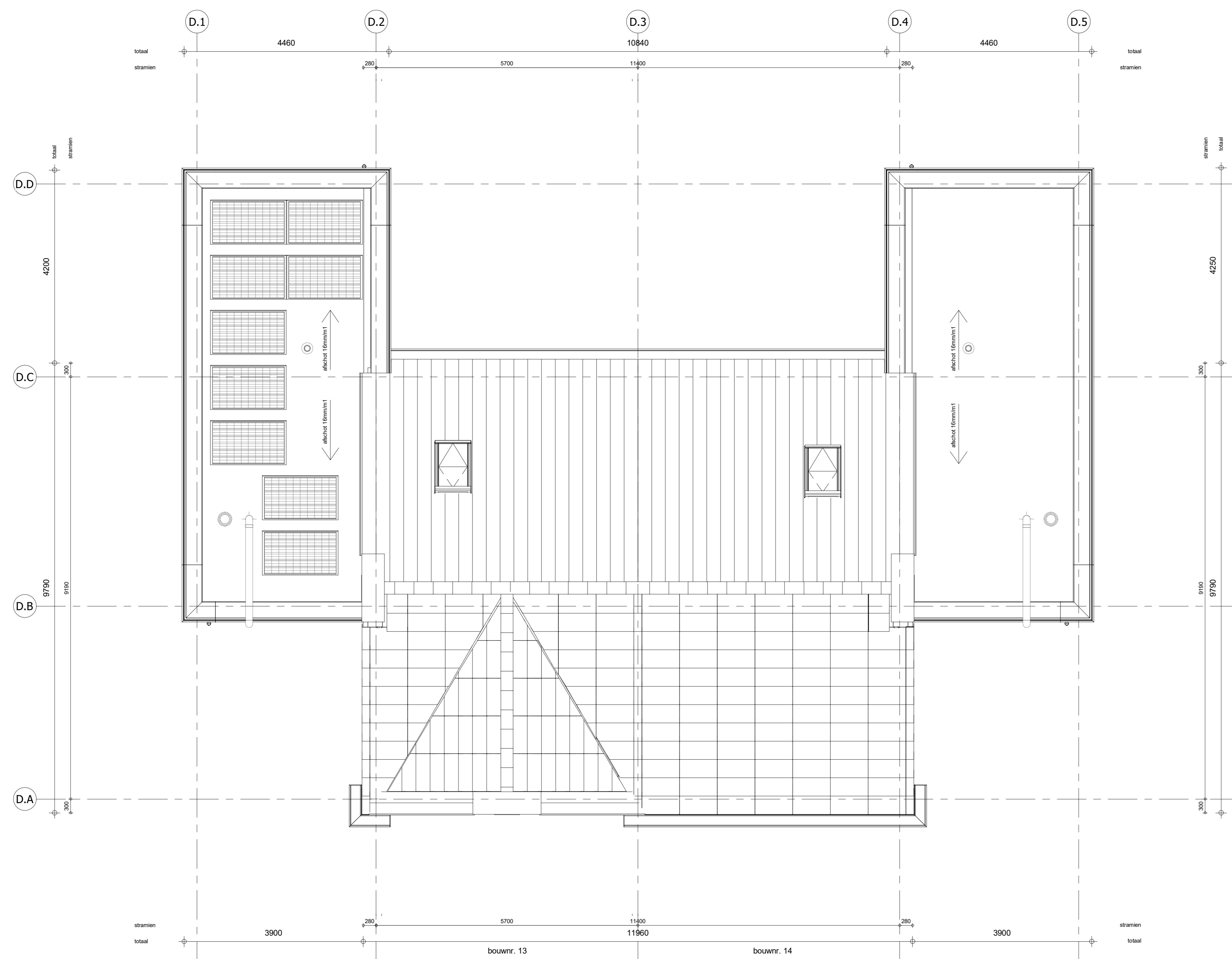
Dakaanzicht 1 : 50
