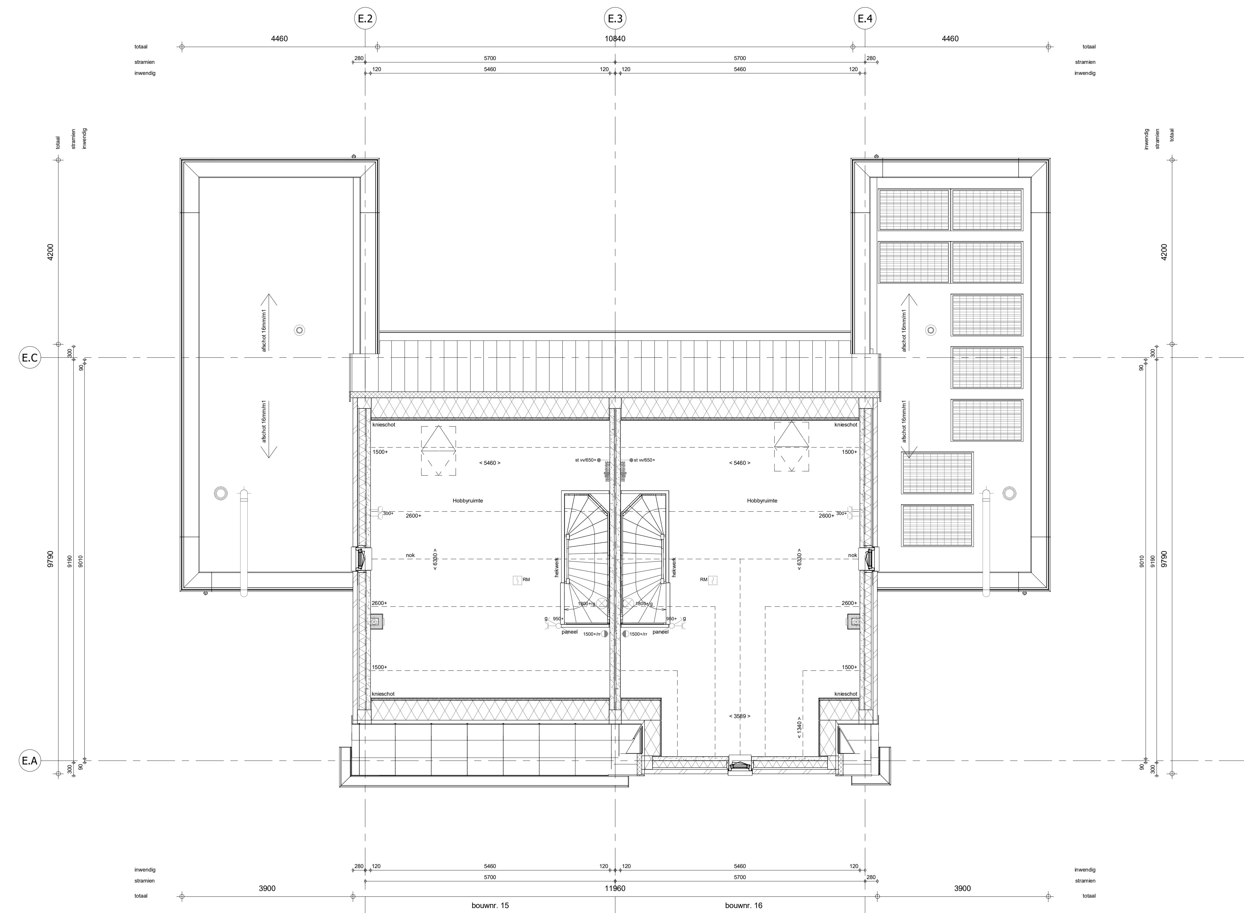
1e verdieping 1 : 50
