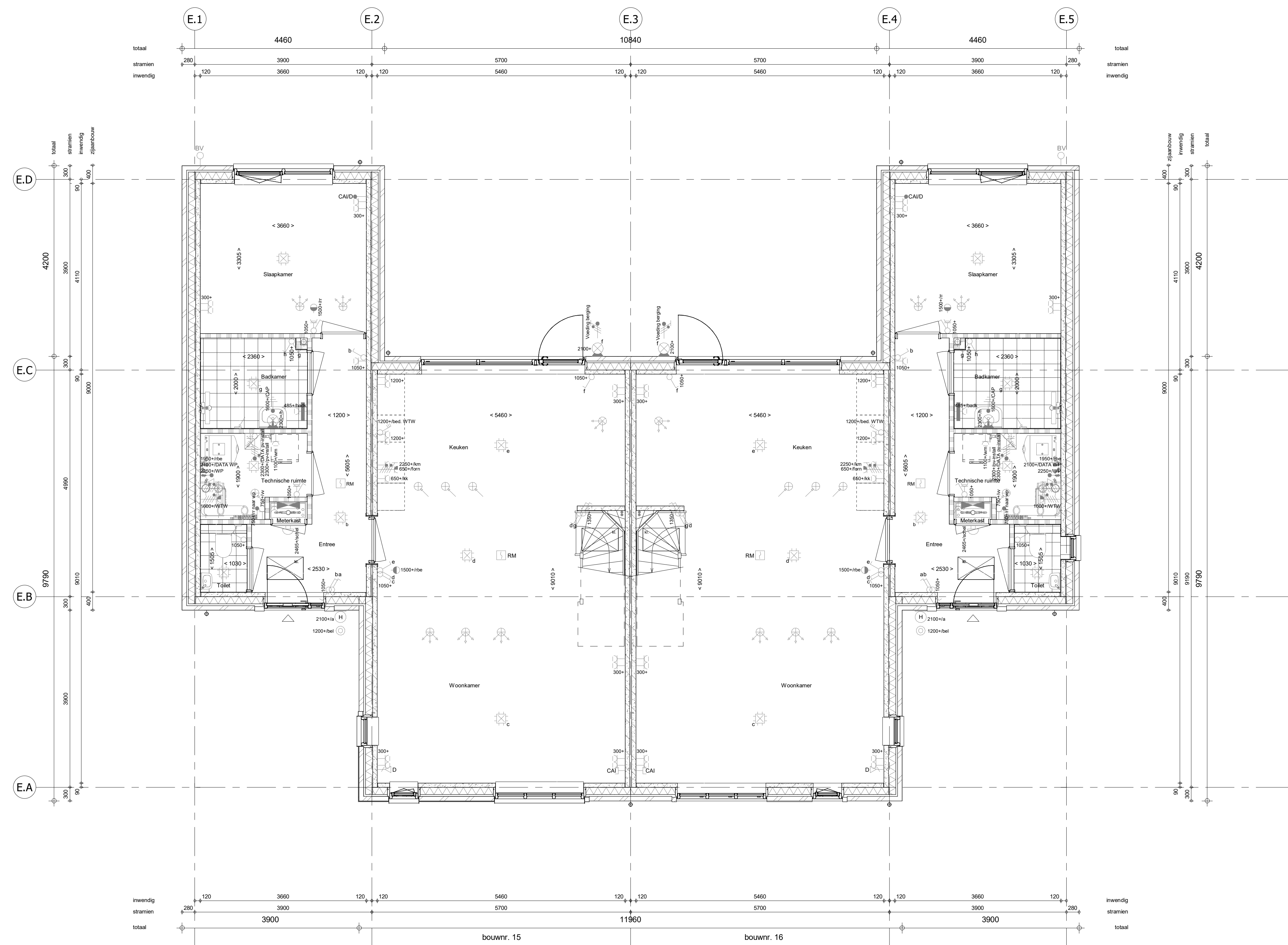
Begane grond 1 : 50
