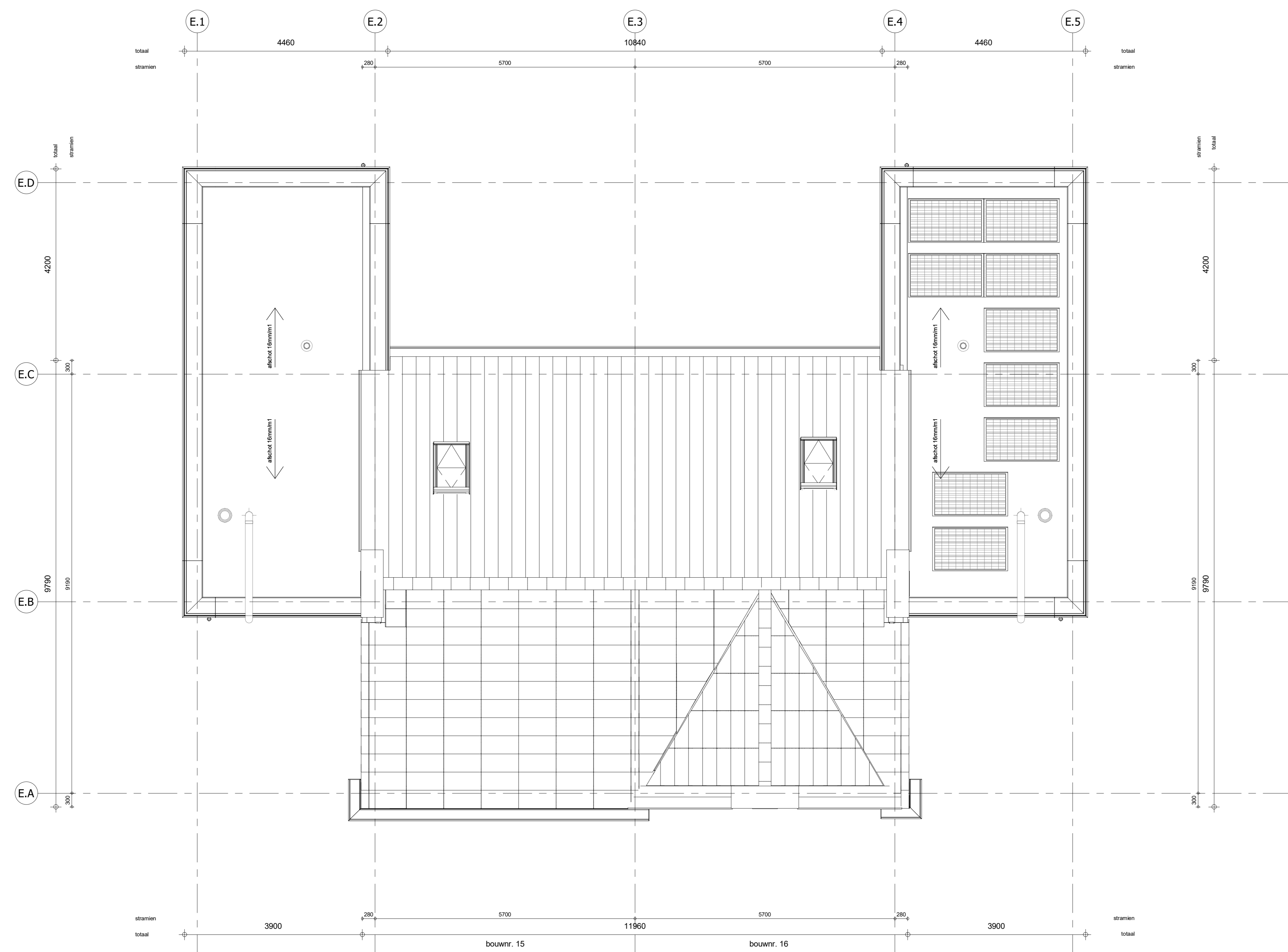
Dakaanzicht 1 : 50
