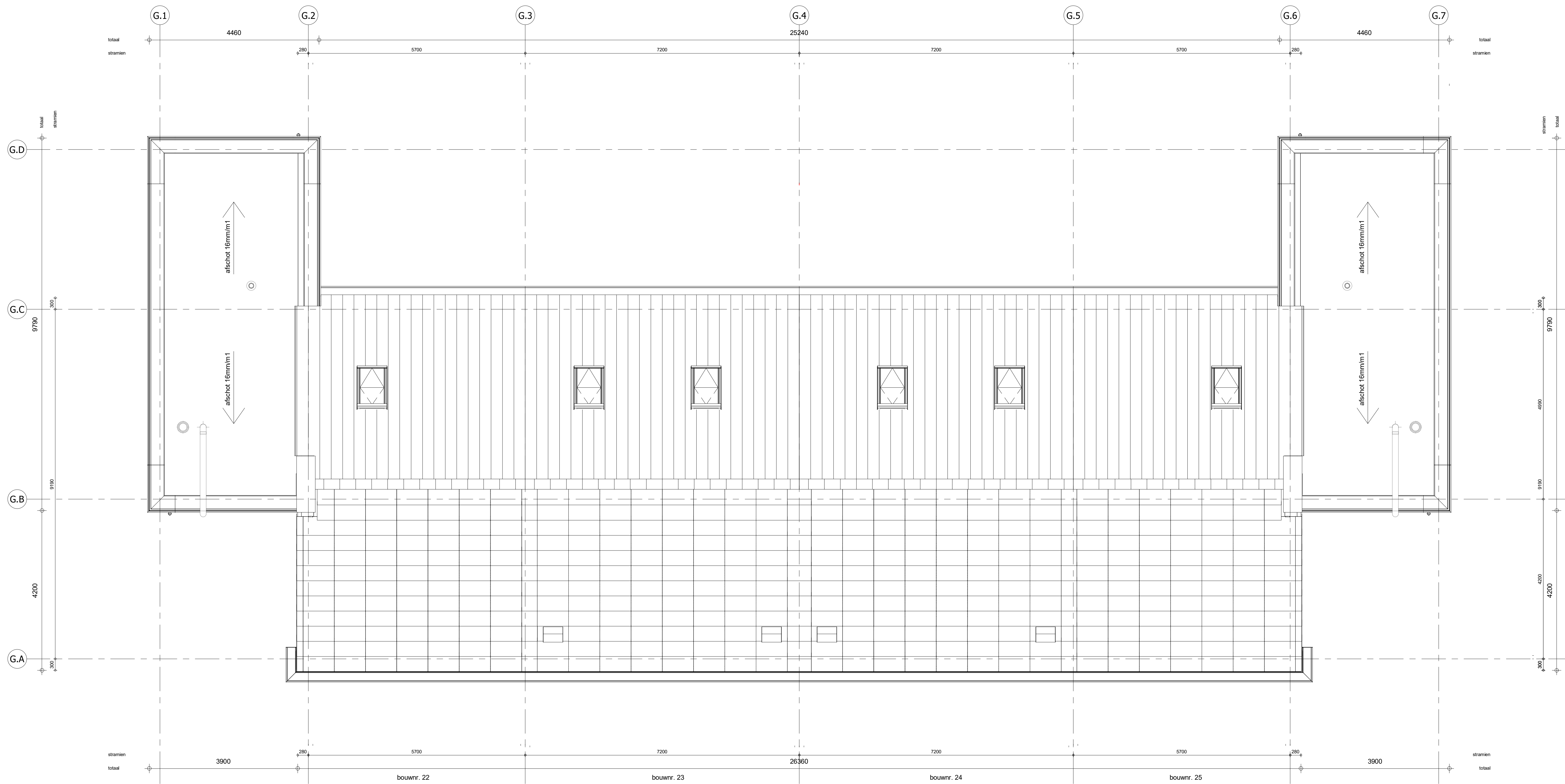
Dakaanzicht 1 : 50
