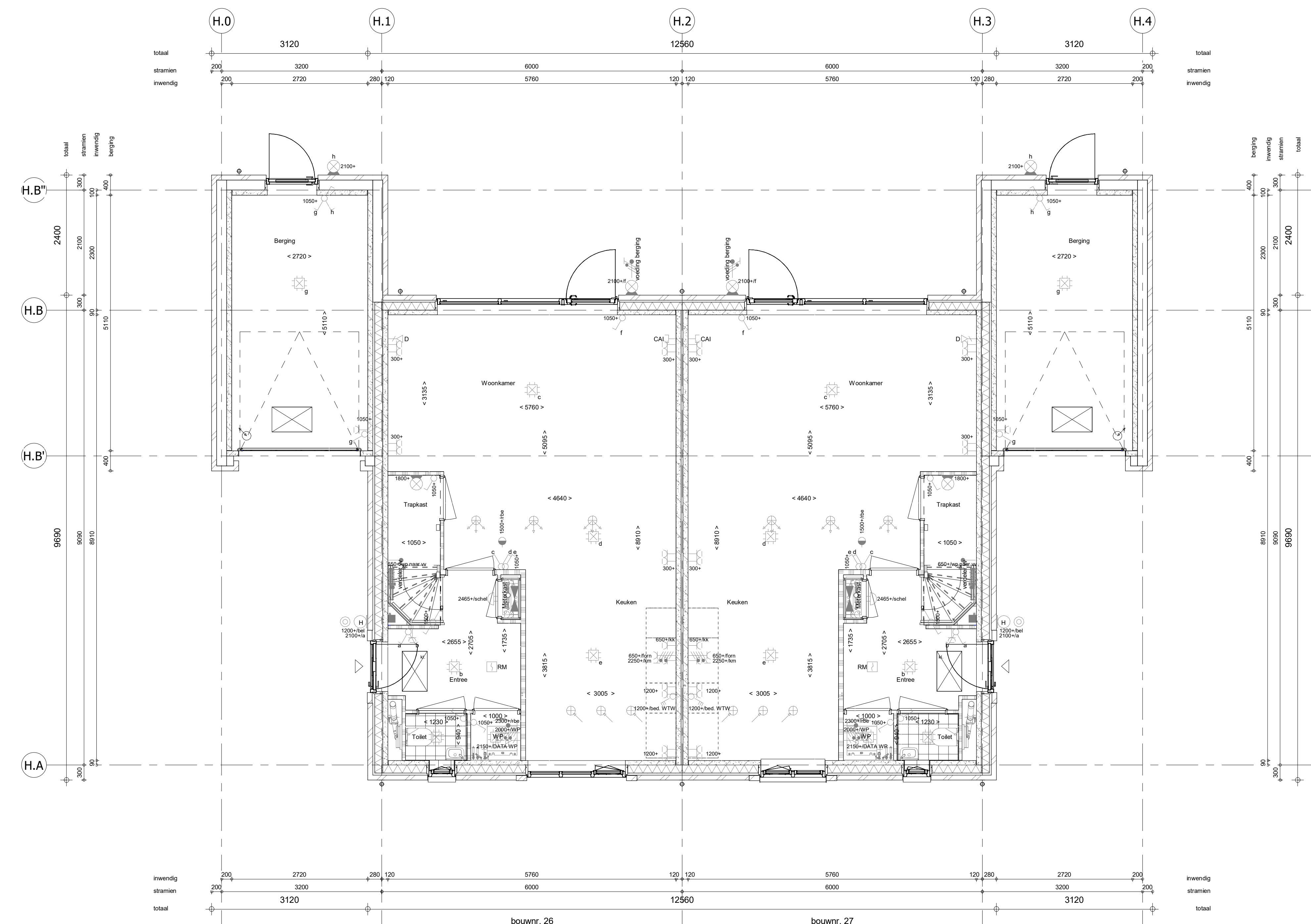
Begane grond 1 : 50
