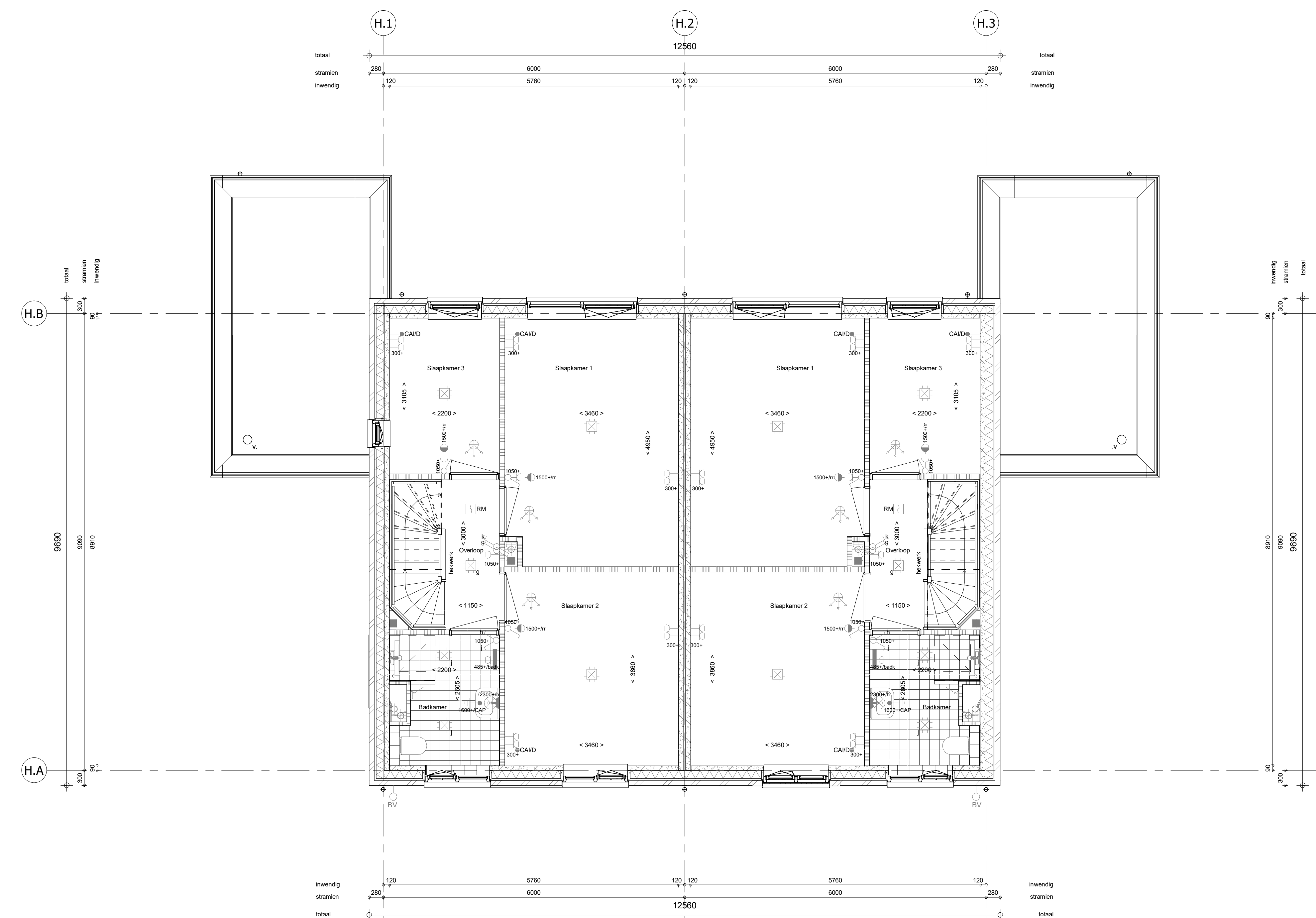
1e verdieping 1 : 50
