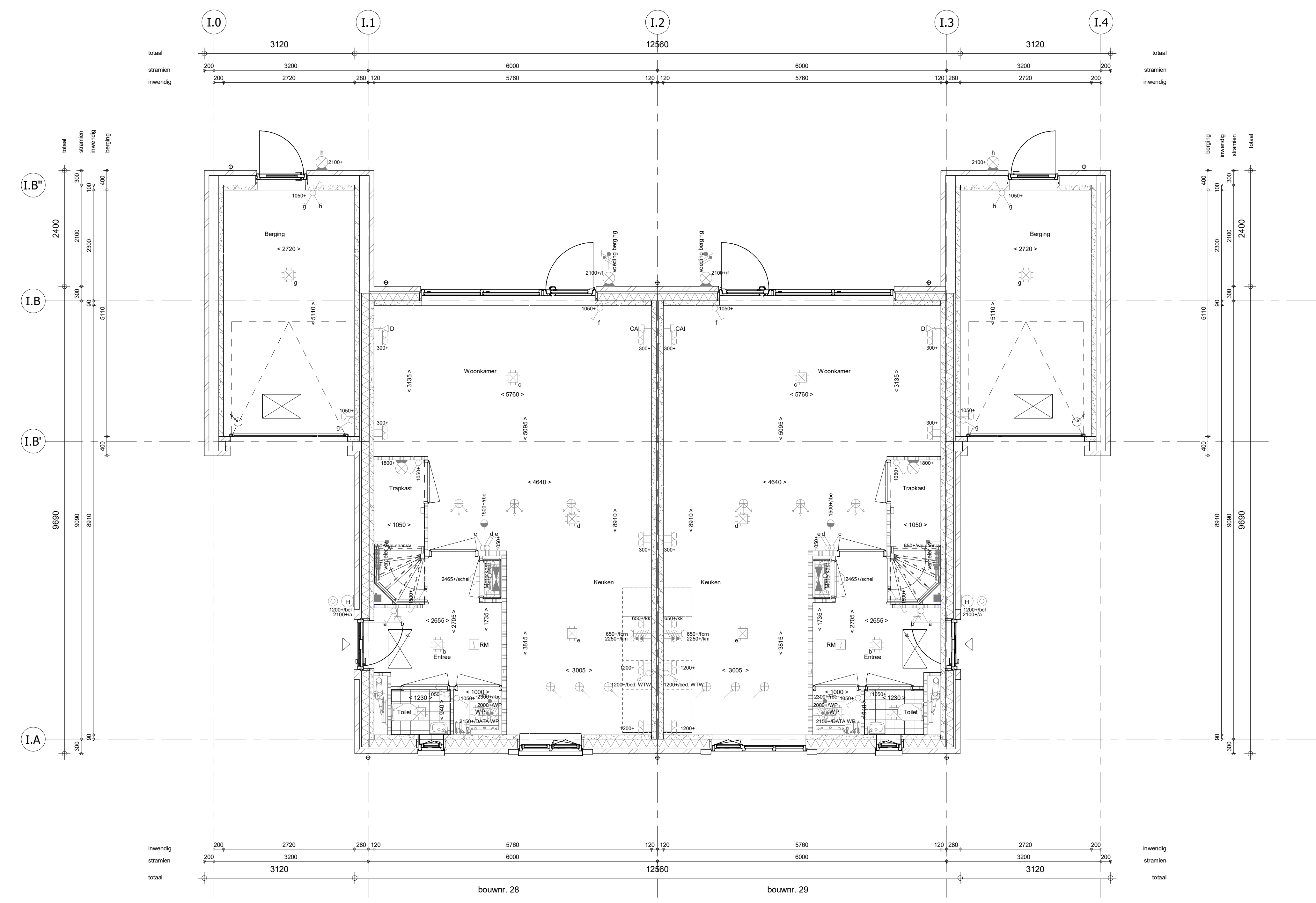
Begane grond 1 : 50
