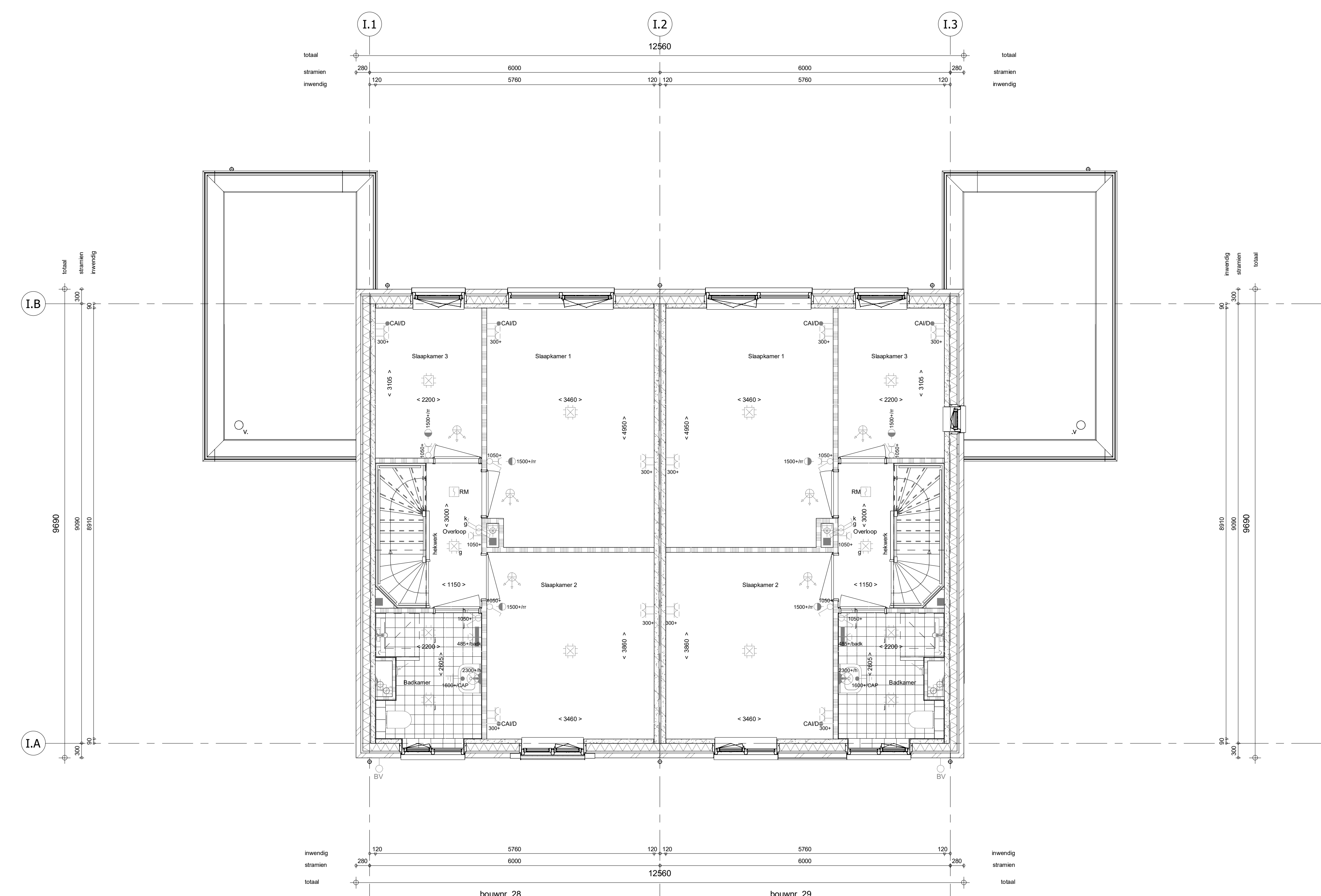
1e verdieping 1 : 50
